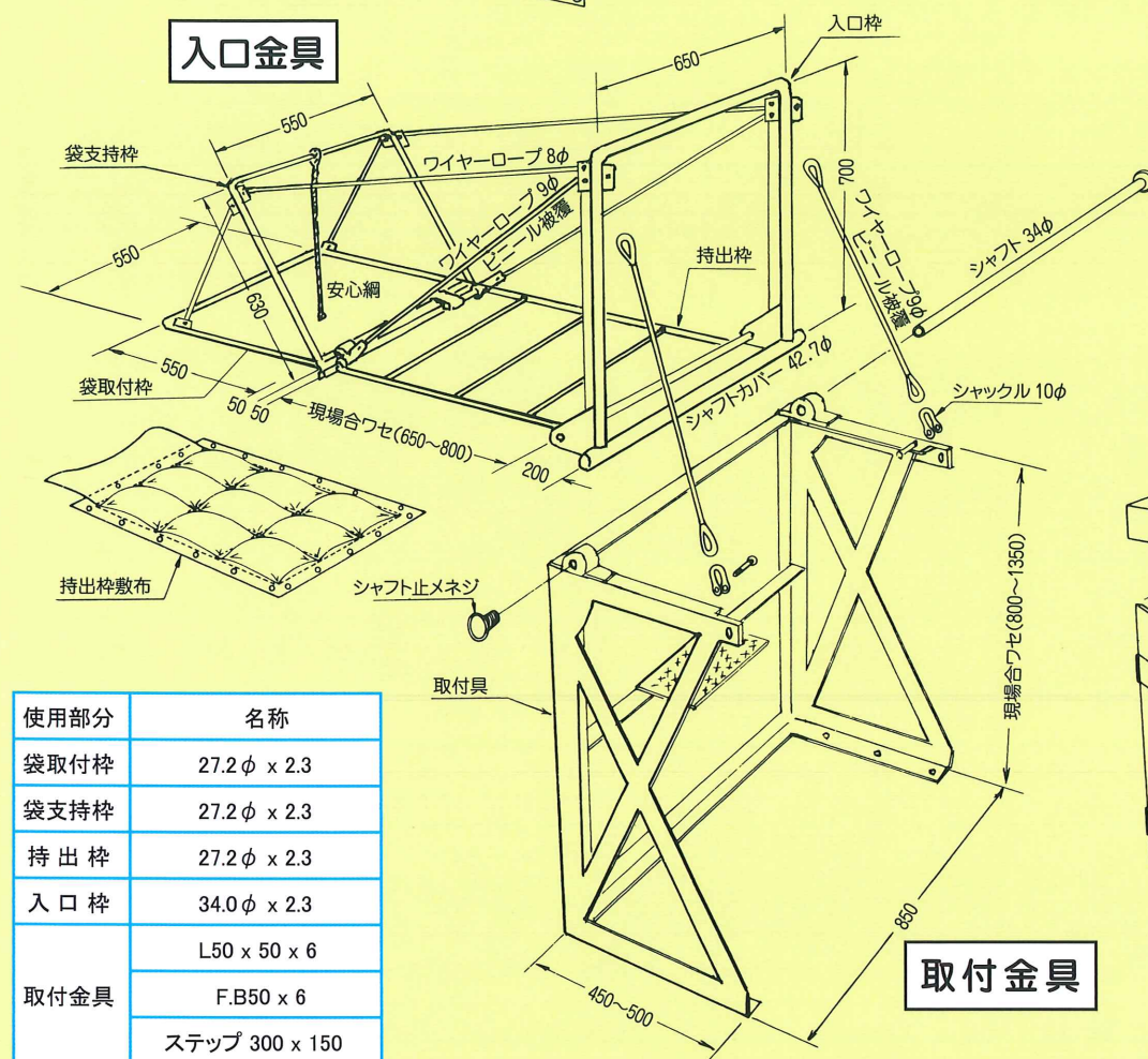
分解型格納箱
